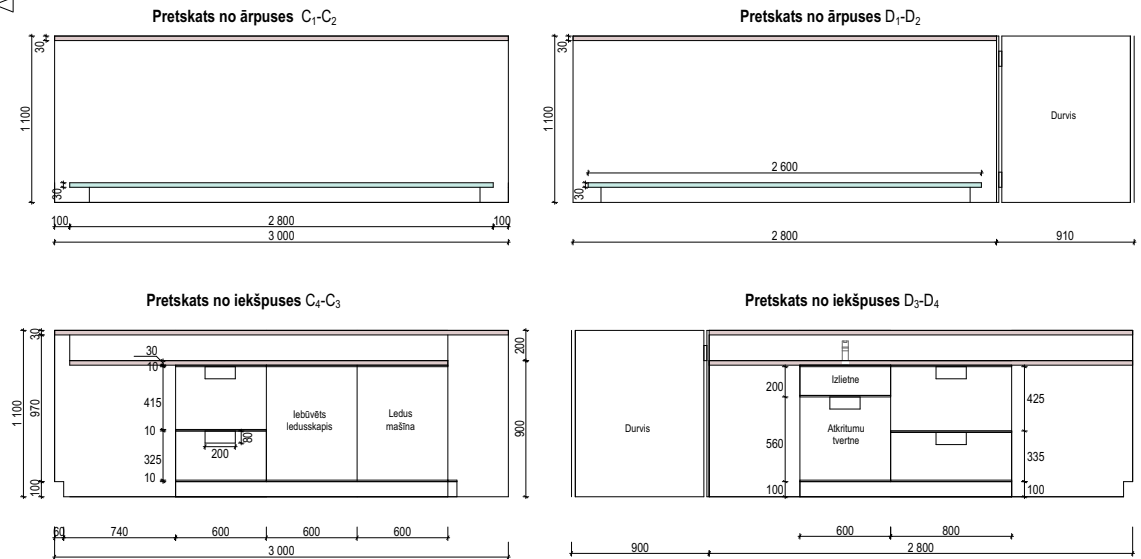
BĀRA LETES GABARĪTRASĒJUMS M1:50
