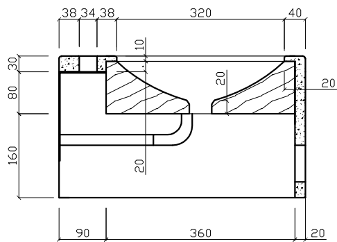
Griezums A - A
